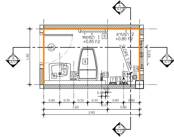
แปลนขยายห้องน้ำ IN SCALE 1 : 50
