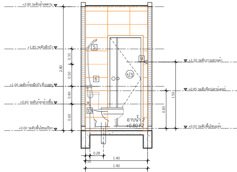
รูปตัดขยายหน้า 2 แนว A IN SCALE 1 : 50
