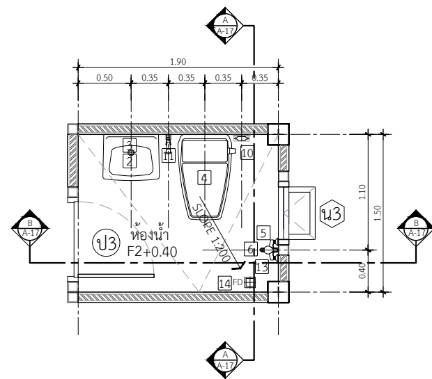
แปลนขยายห้องน้ำ IN SCALE 1 : 50
