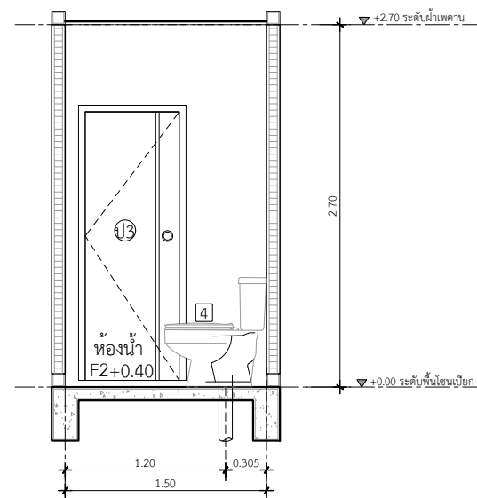
รูปตัดขยายห้องน้ำ 1 แนว A IN SCALE 1 : 50
