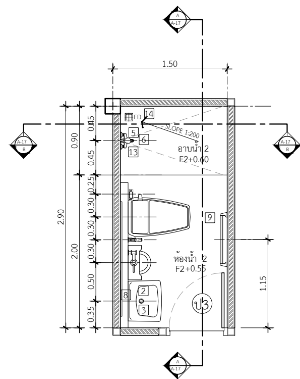
แปลนขยายห้องน้ำ 2 IN SCALE 1 : 50
