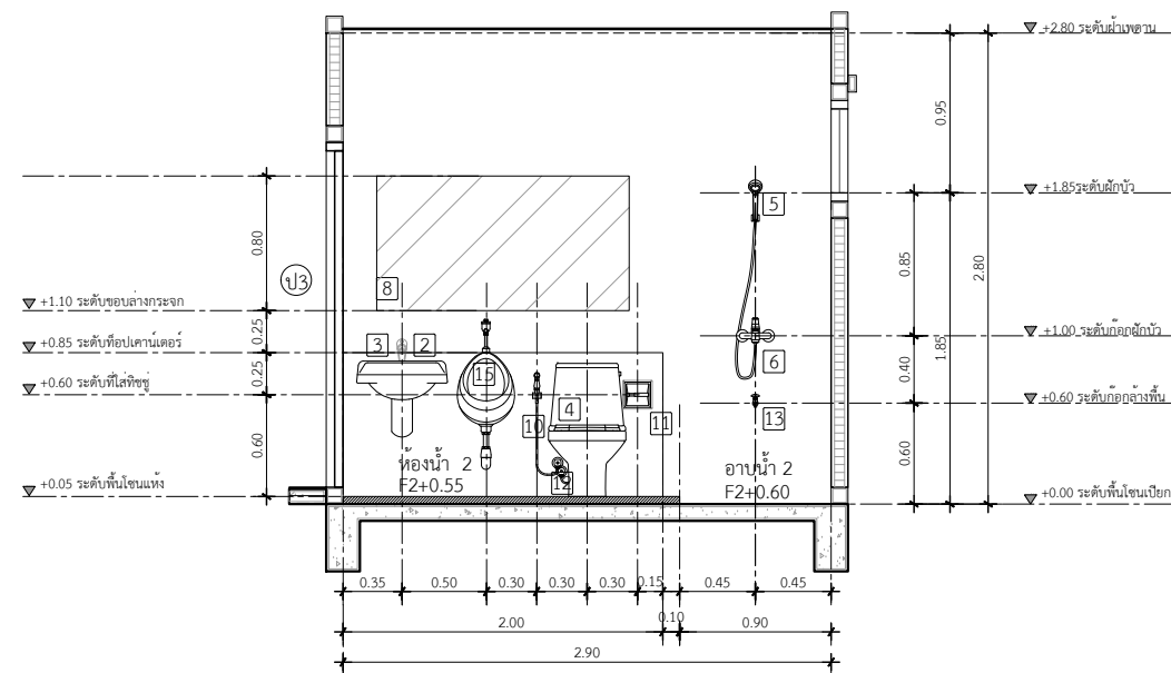
รูปตัดขยายห้องน้ำ 2 แนว A IN SCALE 1 : 50
