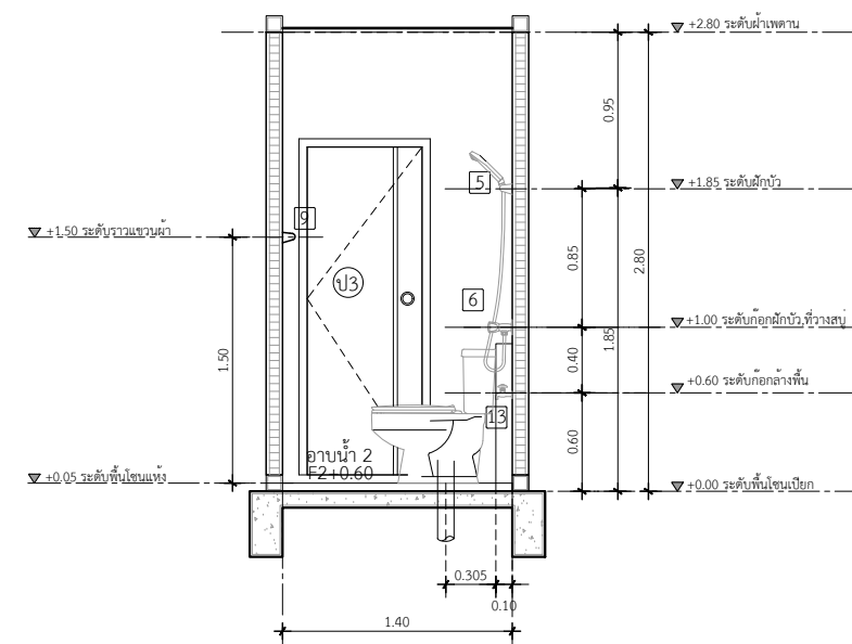
รูปตัดขยายห้องน้ำ 2 แนว B IN SCALE 1 : 50
