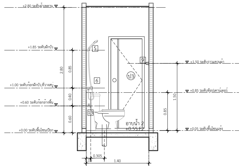
รูปตัดขยายห้องน้ำ 2 แนว A
