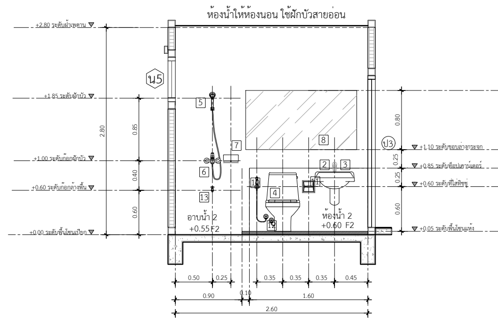
รูปตัดขยายห้องน้ำ 2 แนว B IN SCALE 1 : 50
