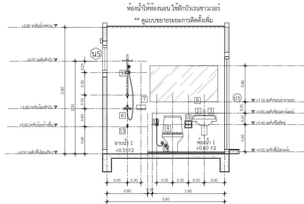
รูปตัดขยายห้องน้ำ 1 แนว B IN SCALE 1 : 50
