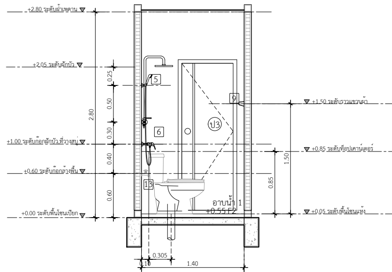
รูปตัดขยายห้องน้ำ 1 แนว A
