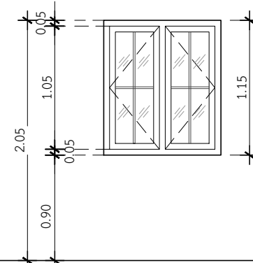
น52 หน้าต่างห้องนอน
