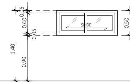
น7 หน้าต่างห้องครัว
