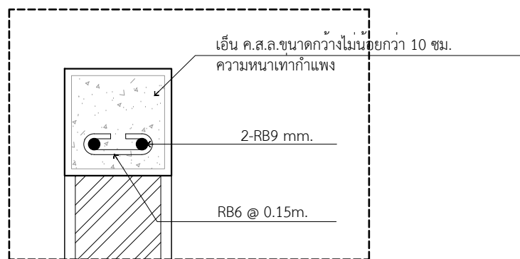
แบบขยายเอ็น ค.ส.ล.
