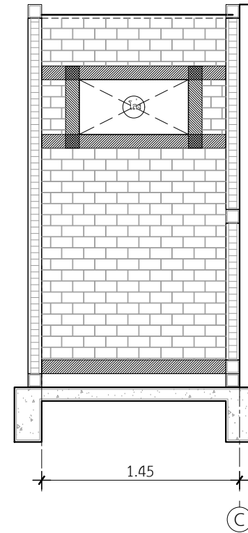
รูปตัดขยายห้องน้ำ 1 แนว B
