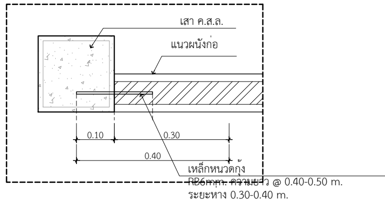
แปลนแบบขยายการฝักทวนดิ่ง
