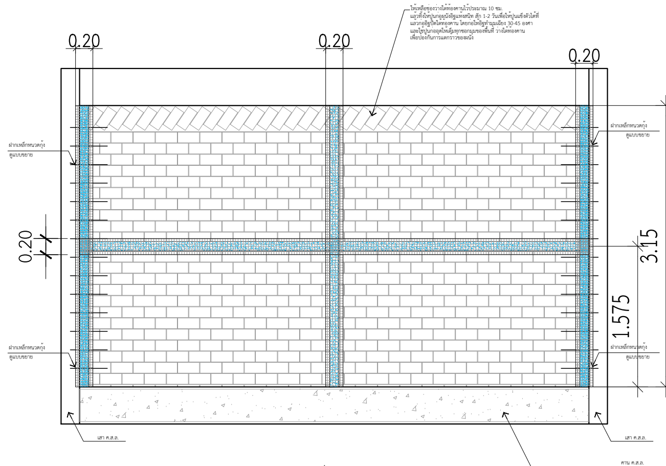
แบบขยายการก่อผนัง (เอ็น ค.ส.ล.)
