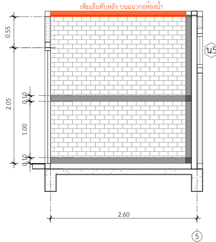
รูปตัดขยายห้องน้ำ 1 แนว A
